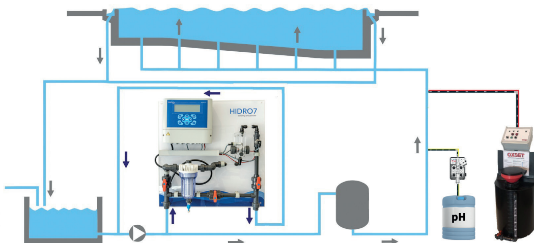
Esquema para piscina
